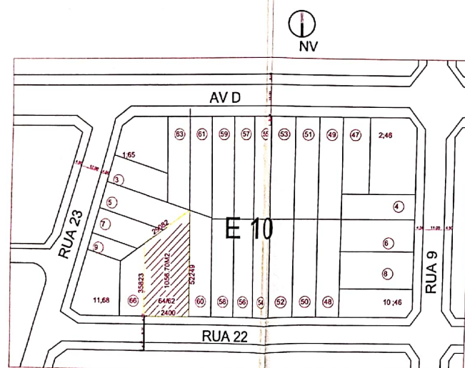
PLANTA DE SITUAÇÃO REMEMBRADA esc. 1:1000
