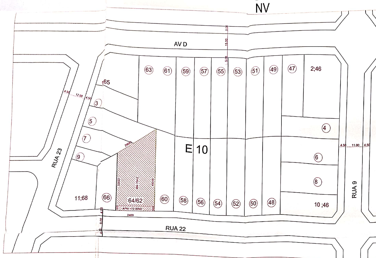
REMANEJAMENTO PROPOSTO ESC.:1:500
