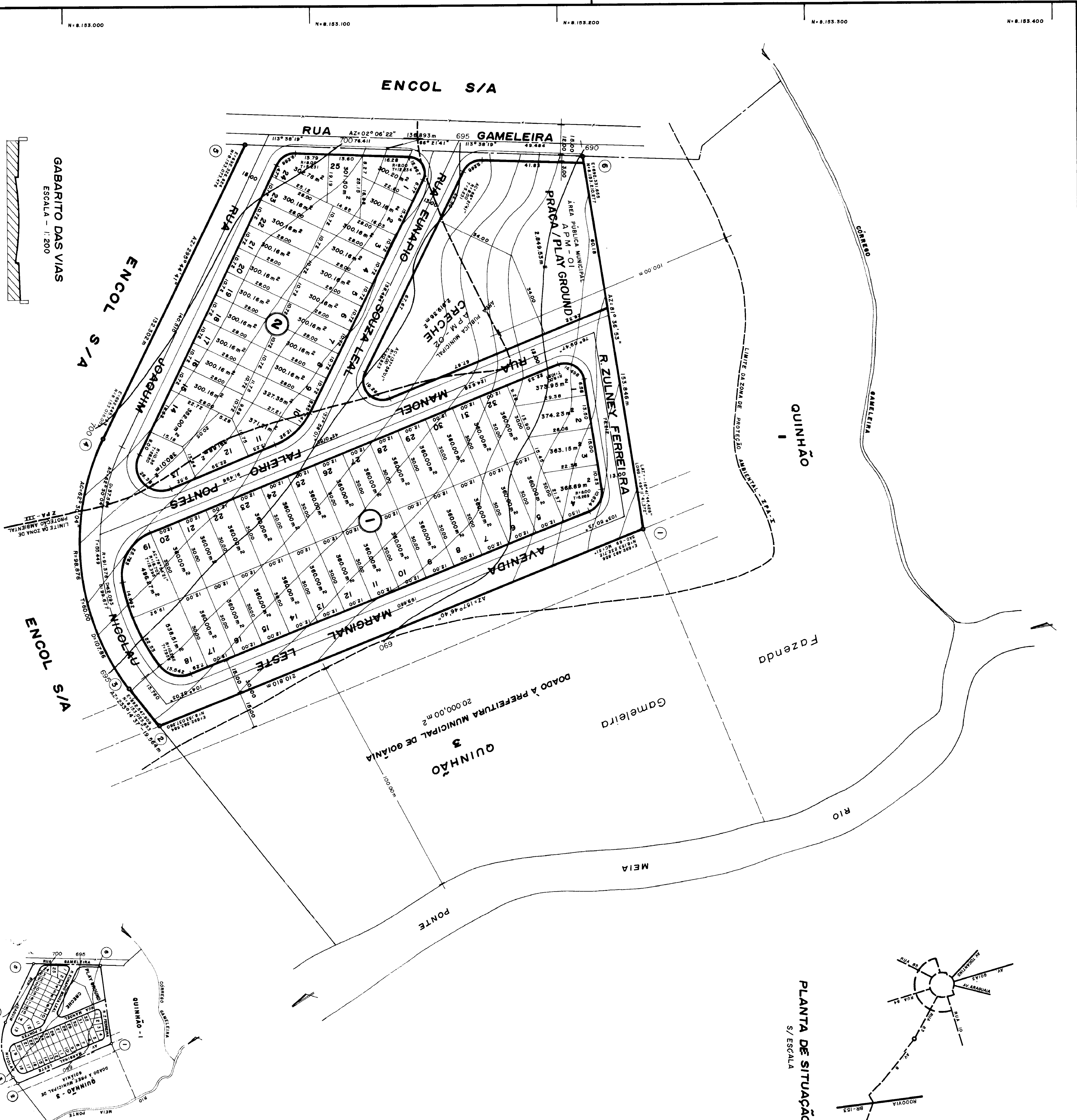
PLANTA DE SITUAÇÃO S/ ESCALA
