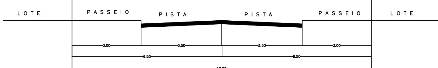
SEÇÃO TRANSVERSAL DAS VIAS DE 13,00 METROS – ESCALA 1/100
