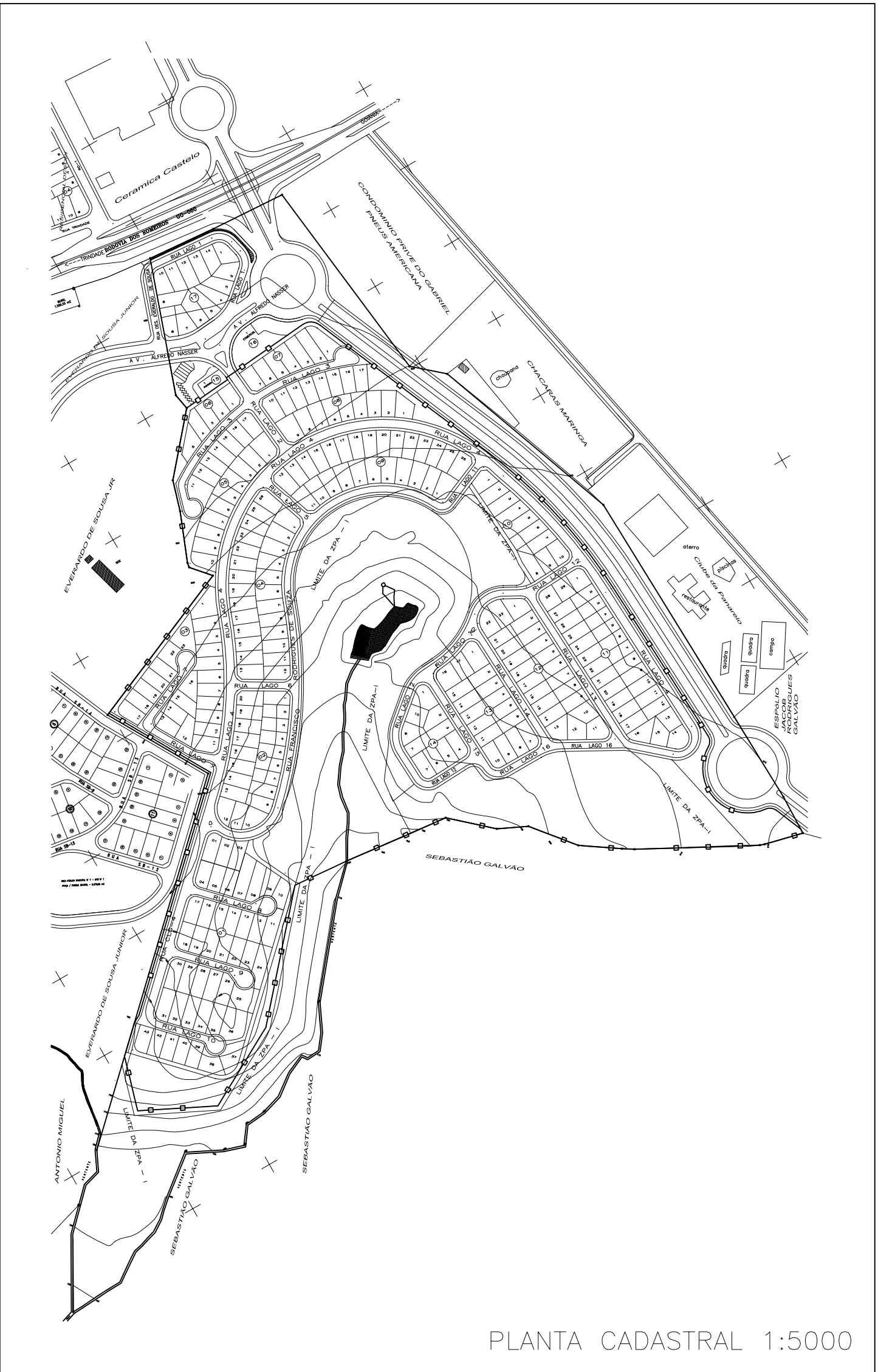
PLANTA CADASTRAL 1:5000
