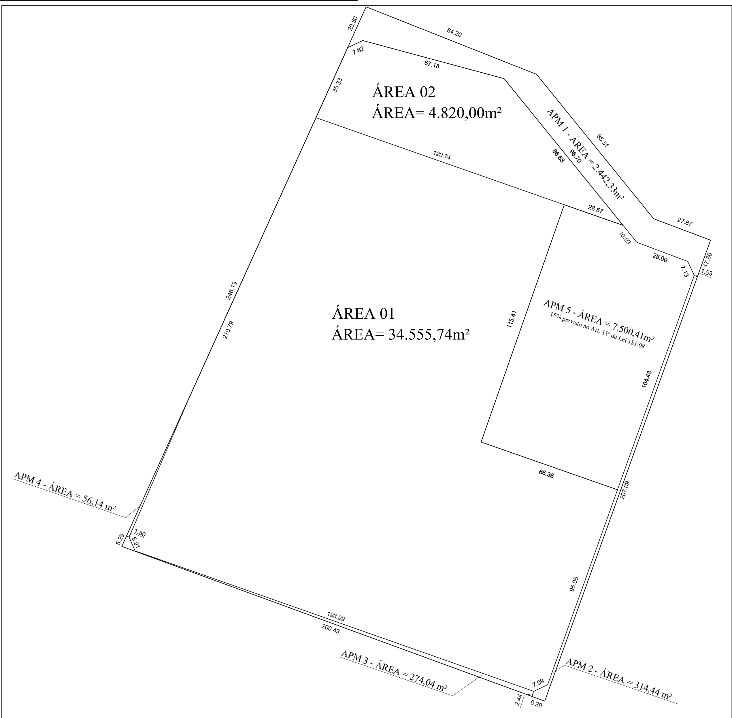
DESMEMBRAMENTO PROPOSTO ESCALA 1:1000
