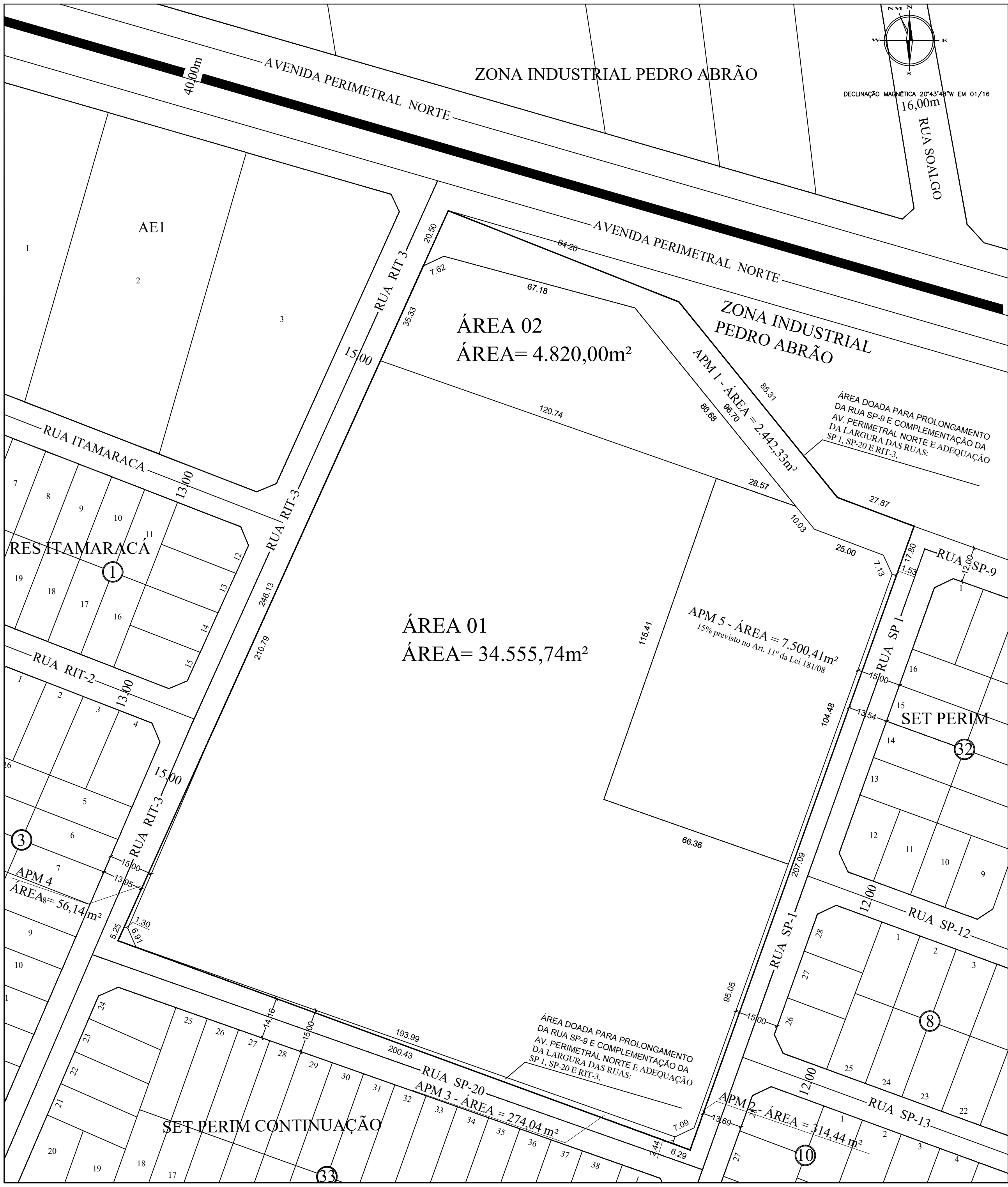
SITUAÇÃO APÓS DESMEMBRAMENTO ESCALA 1:1000
