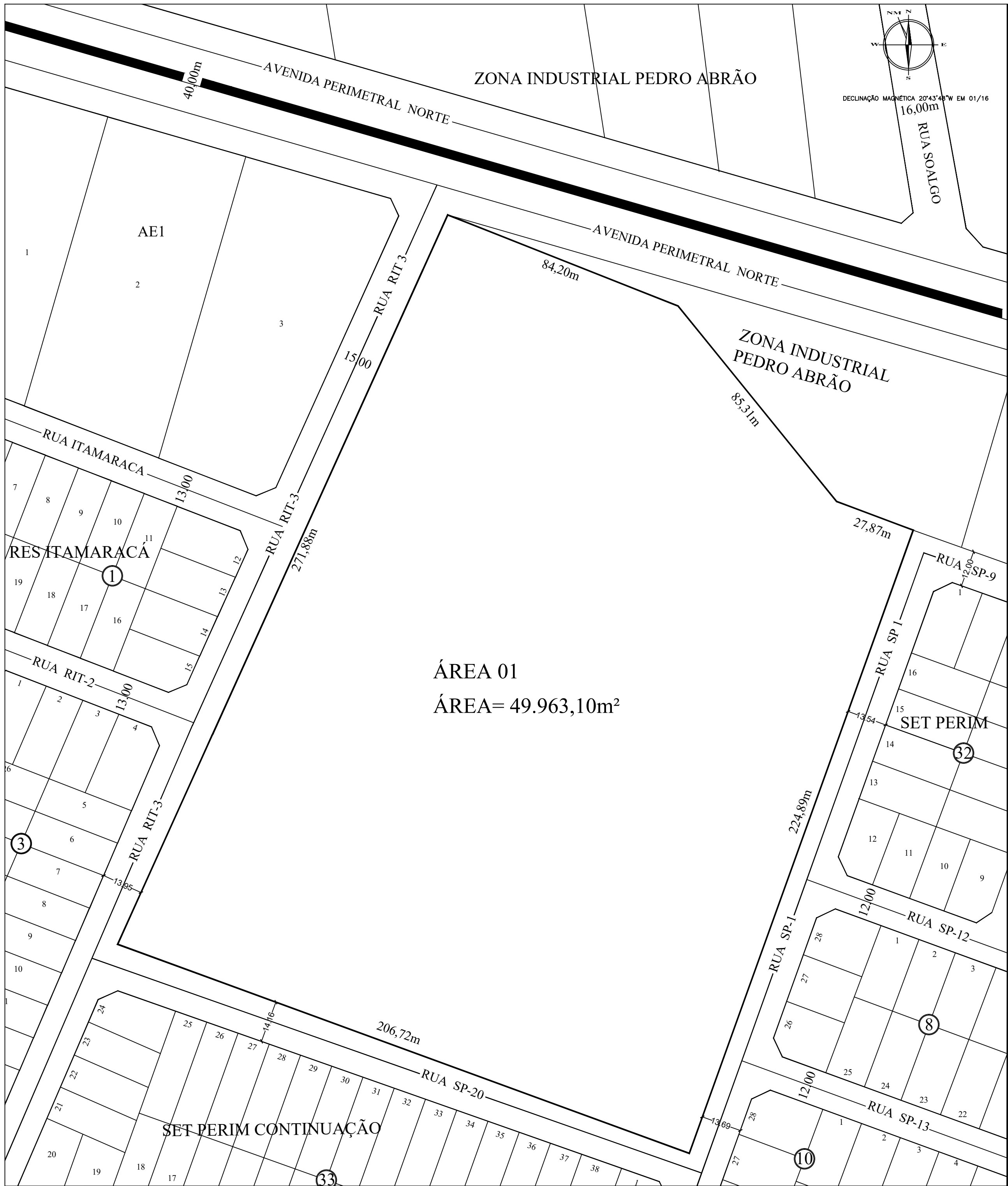
SITUAÇÃO ATUAL ESCALA 1:1000
