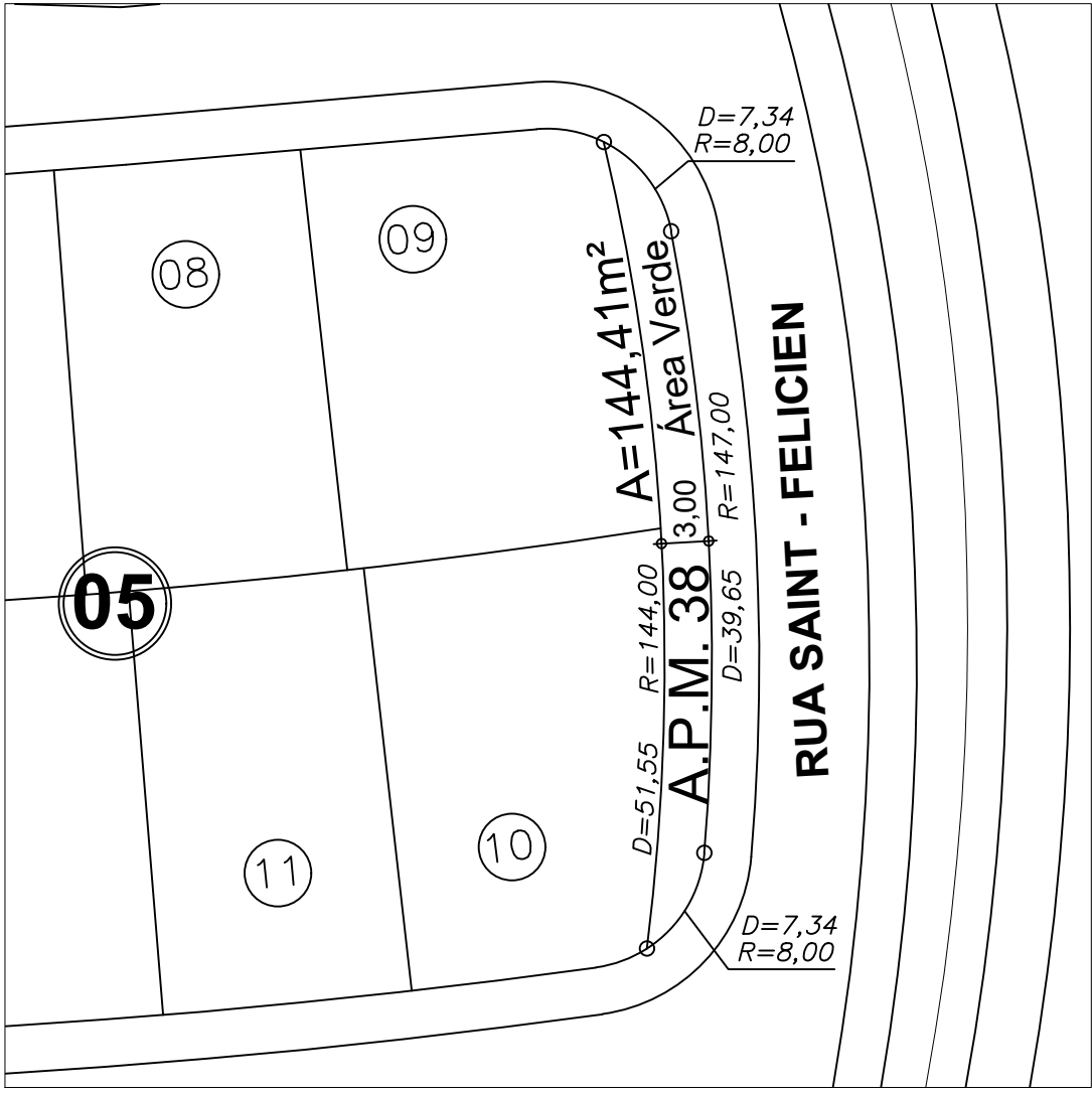
DETALHE DA A.P.M.V. 38 Esc: 1:500
