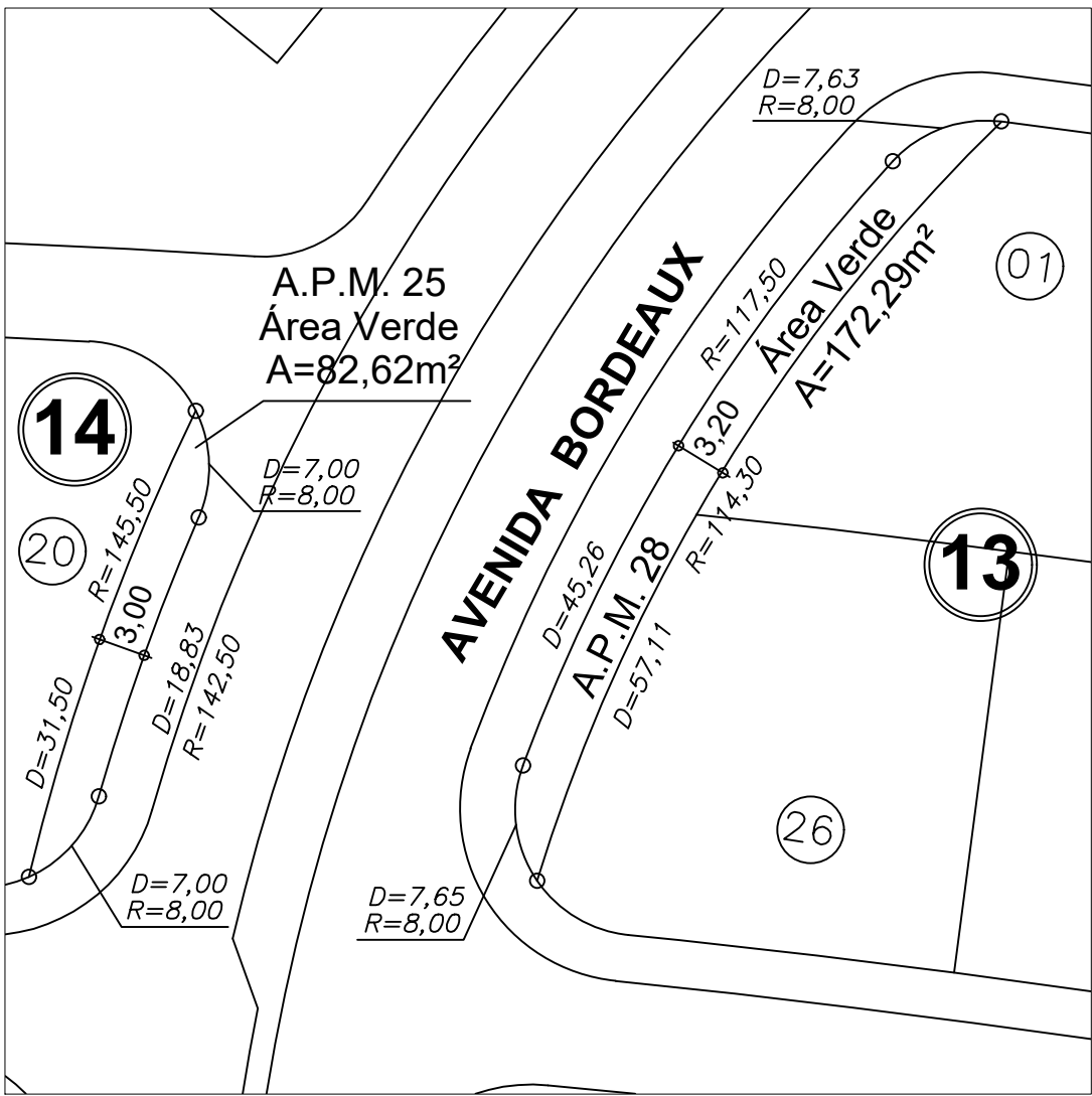
DETALHE DA A.P.M.V. 25 e A.P.M.V. 28 Esc: 1:500
