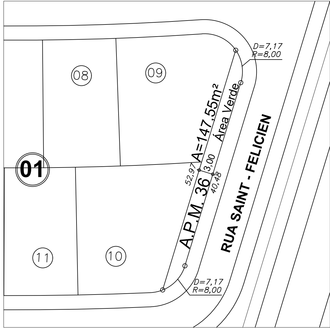
DETALHE DA A.P.M.V. 36 Esc: 1:500
