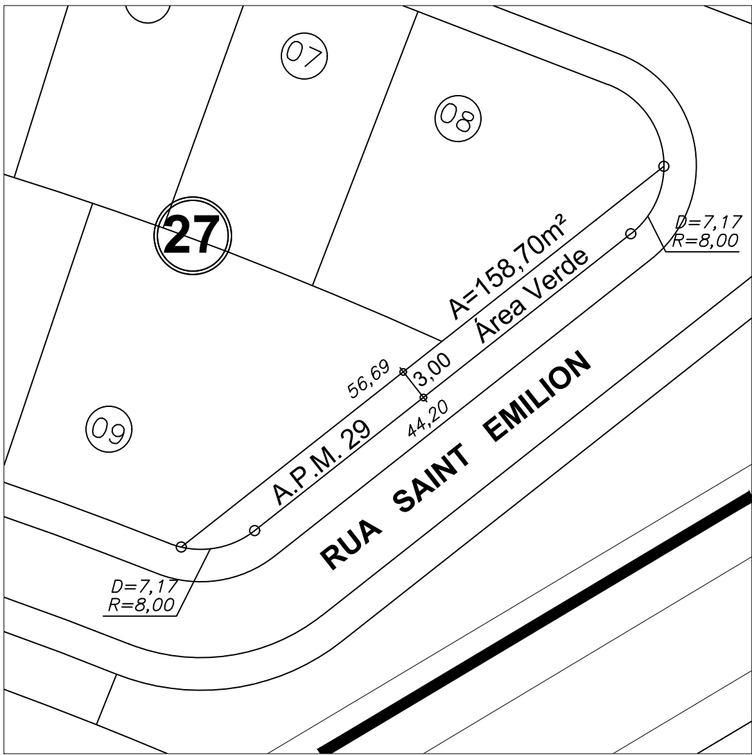
DETALHE DA A.P.M.V. 29 Esc: 1:500
