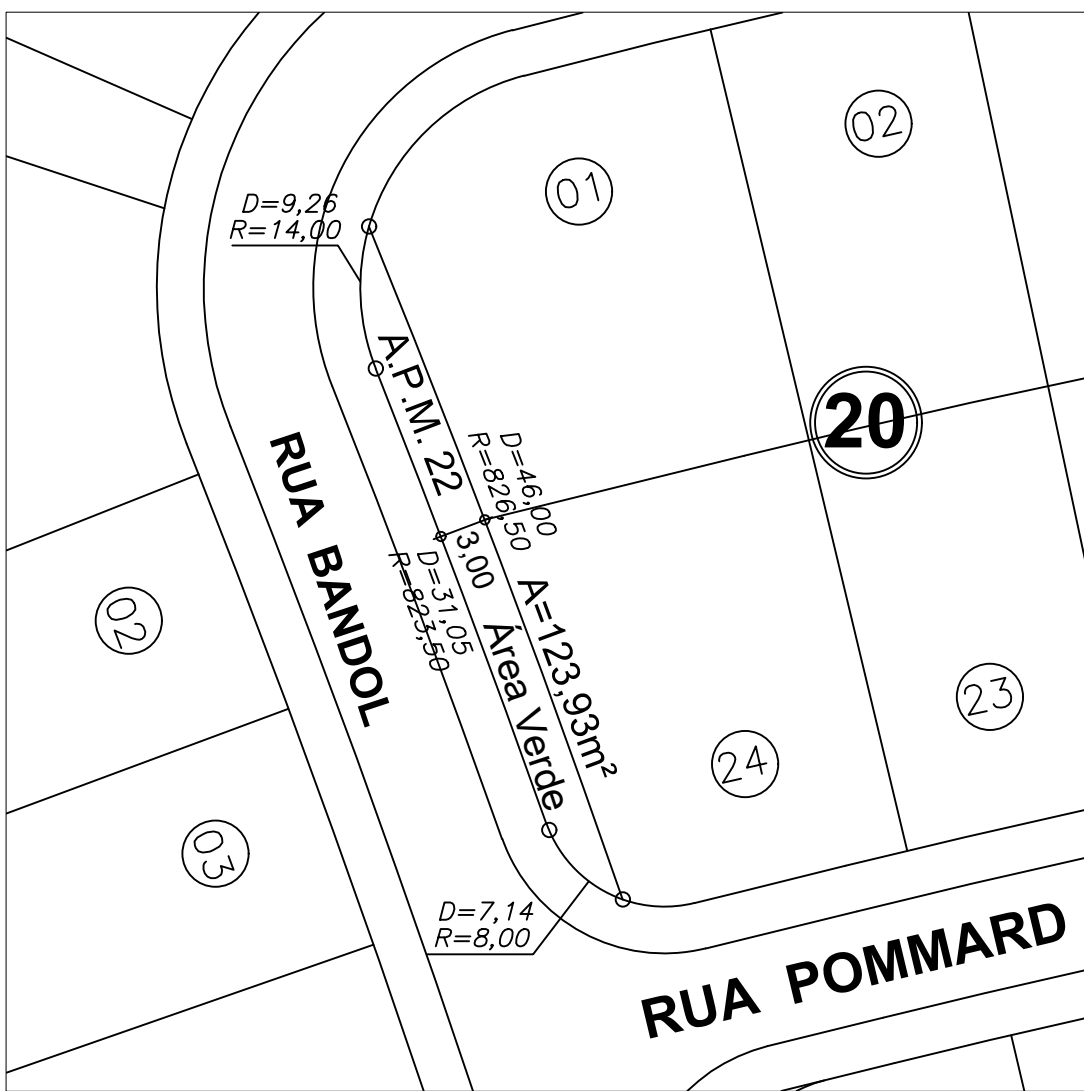
DETALHE DA A.P.M.V. 22 Esc: 1:500
