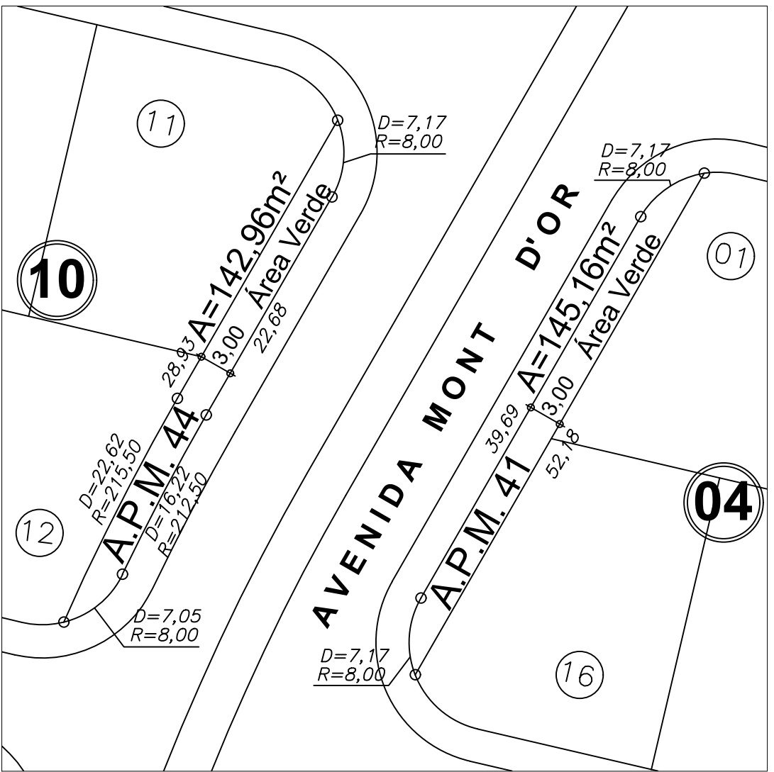
DETALHE DA A.P.M.V. 41 e A.P.M.V. 44 Esc: 1:500
