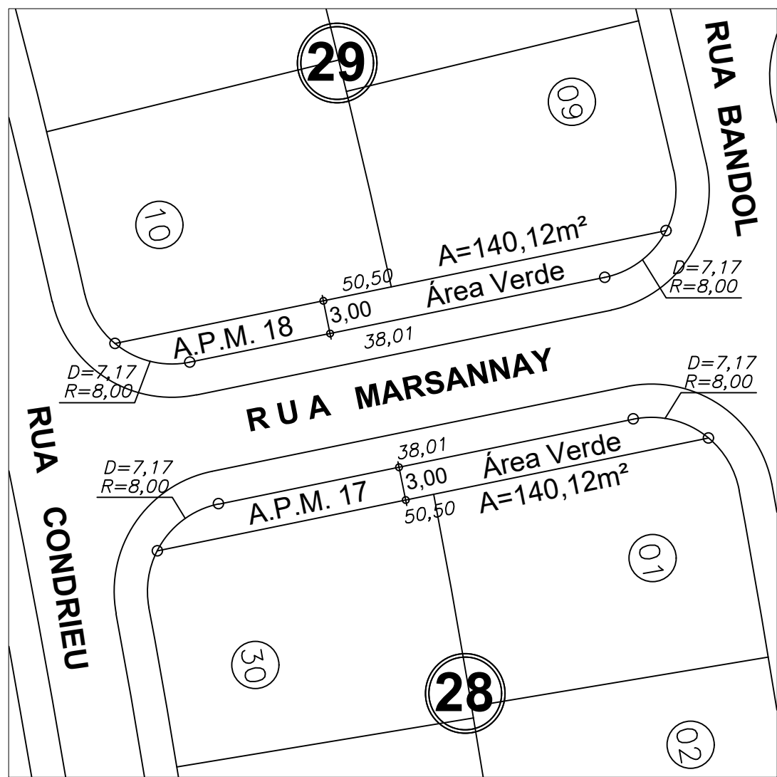
DETALHE DA A.P.M.V. 17 e A.P.M.V. 18 Esc: 1:500
