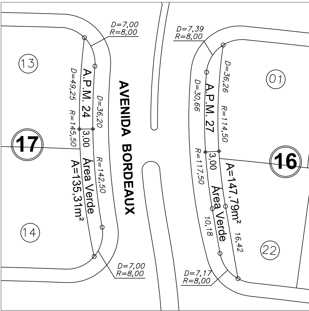
DETALHE DA A.P.M.V. 24 e A.P.M.V. 27 Esc: 1:500
