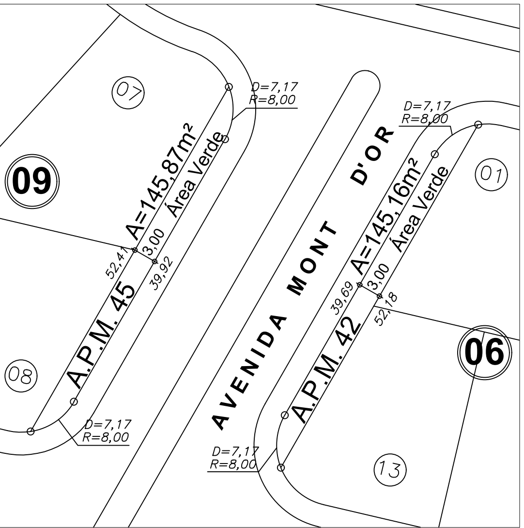
DETALHE DA A.P.M.V. 42 e A.P.M.V. 45 Esc: 1:500
