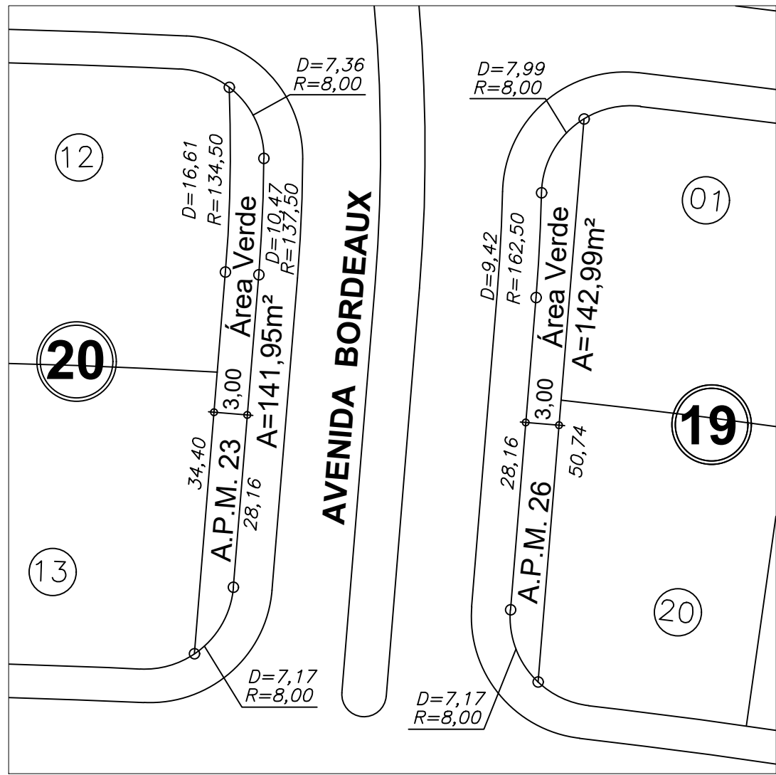
DETALHE DA A.P.M.V. 23 e A.P.M.V. 26 Esc: 1:500
