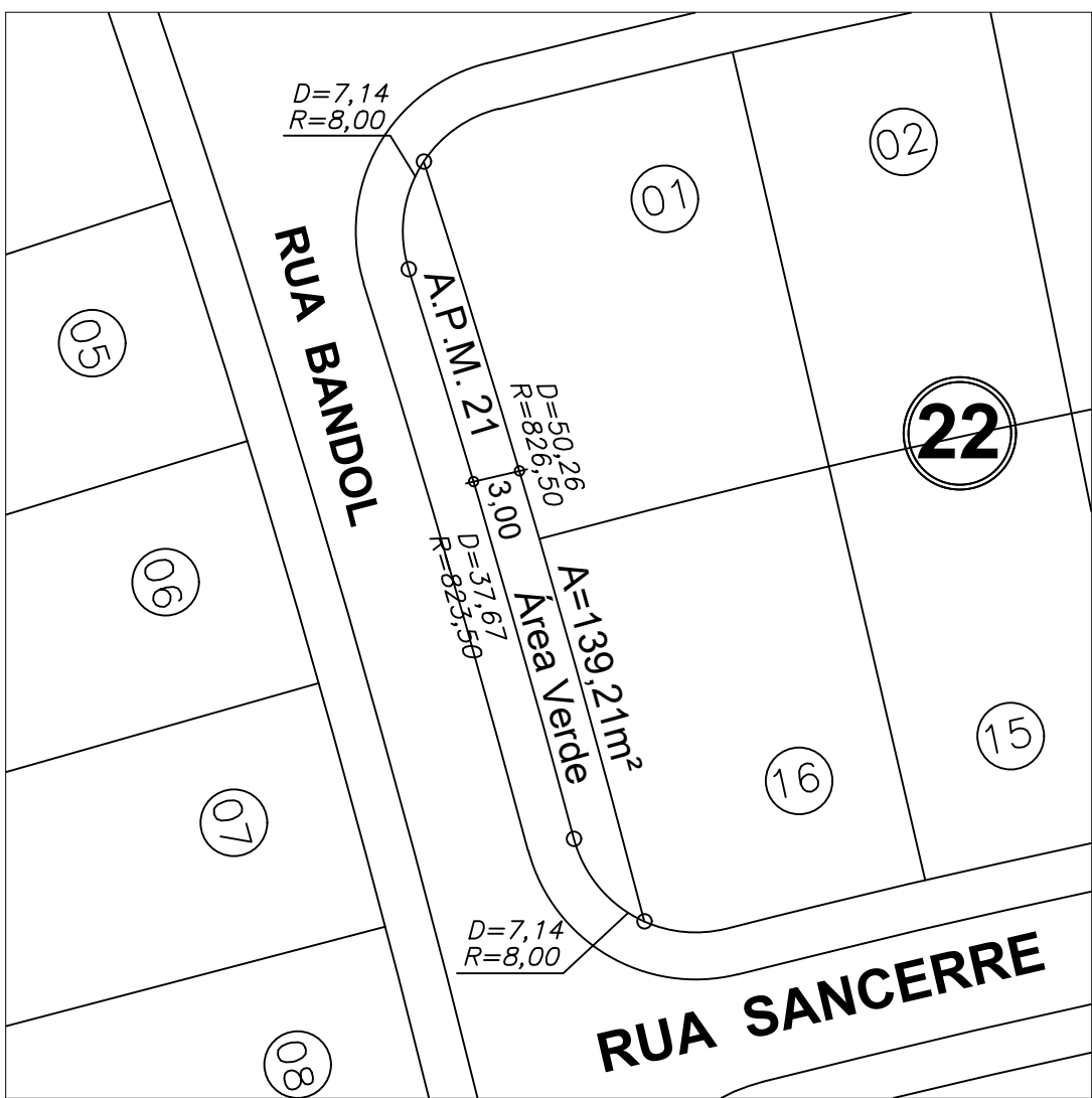
DETALHE DA A.P.M.V. 21 Esc: 1:500
