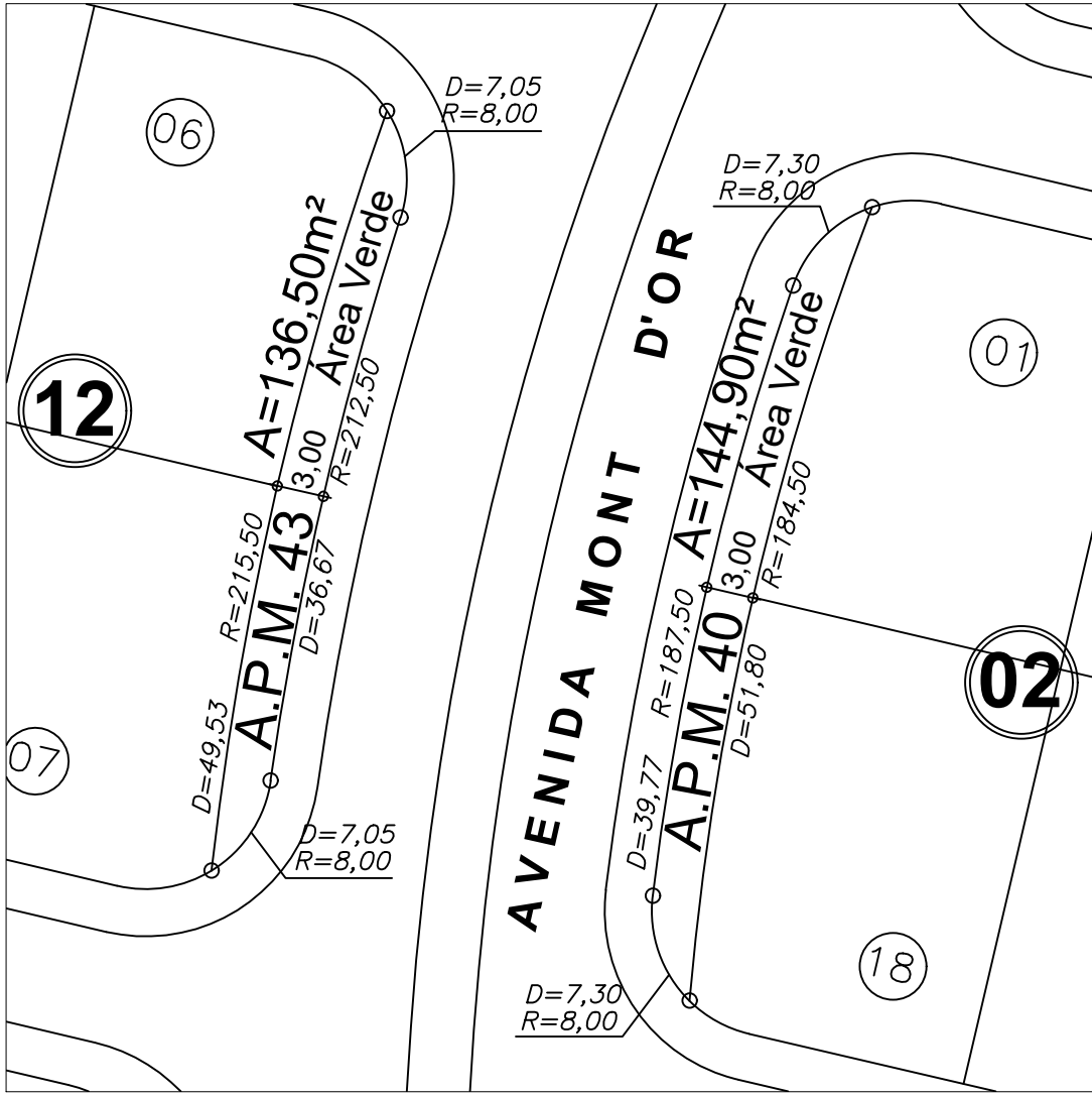
DETALHE DA A.P.M.V. 40 e A.P.M.V. 43 Esc: 1:500
