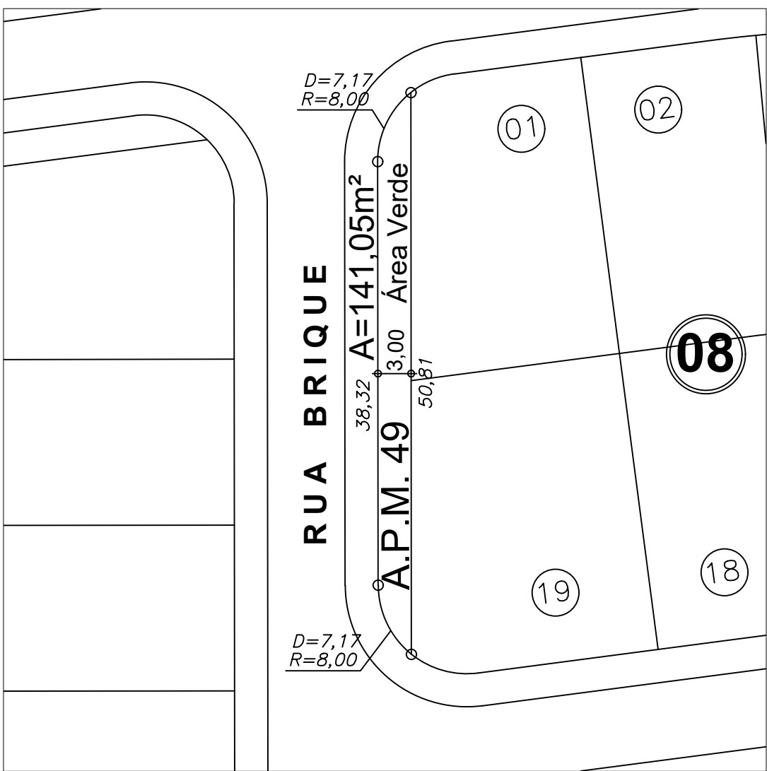
DETALHE DA A.P.M.V. 49 Esc: 1:500
