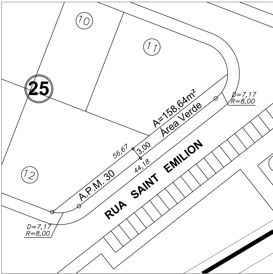
DETALHE DA A.P.M.V. 30 Esc: 1:500
