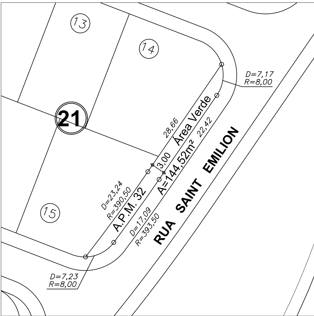
DETALHE DA A.P.M.V. 32 Esc: 1:500
