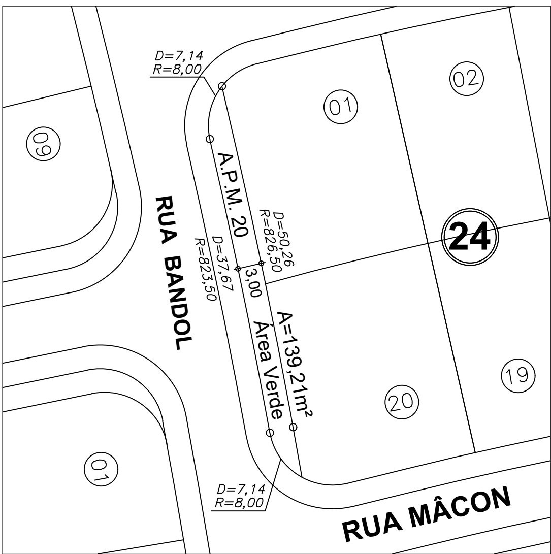
DETALHE DA A.P.M.V. 20 Esc: 1:500
