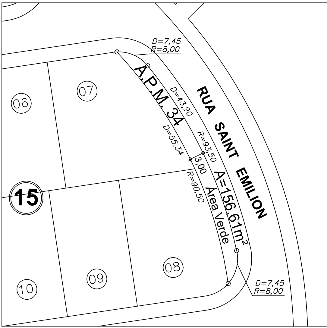
DETALHE DA A.P.M.V. 34 Esc: 1:500
