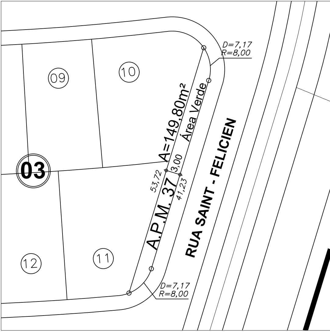
DETALHE DA A.P.M.V. 37 Esc: 1:500
