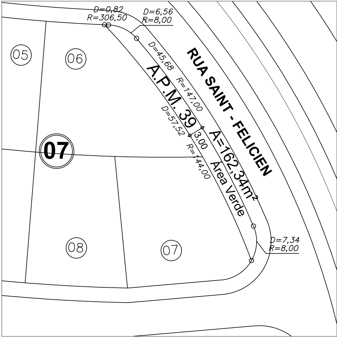
DETALHE DA A.P.M.V. 39 Esc: 1:500
