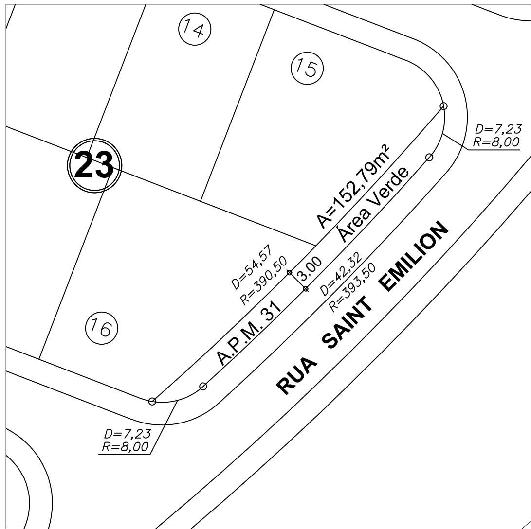
DETALHE DA A.P.M.V. 31 Esc: 1:500
