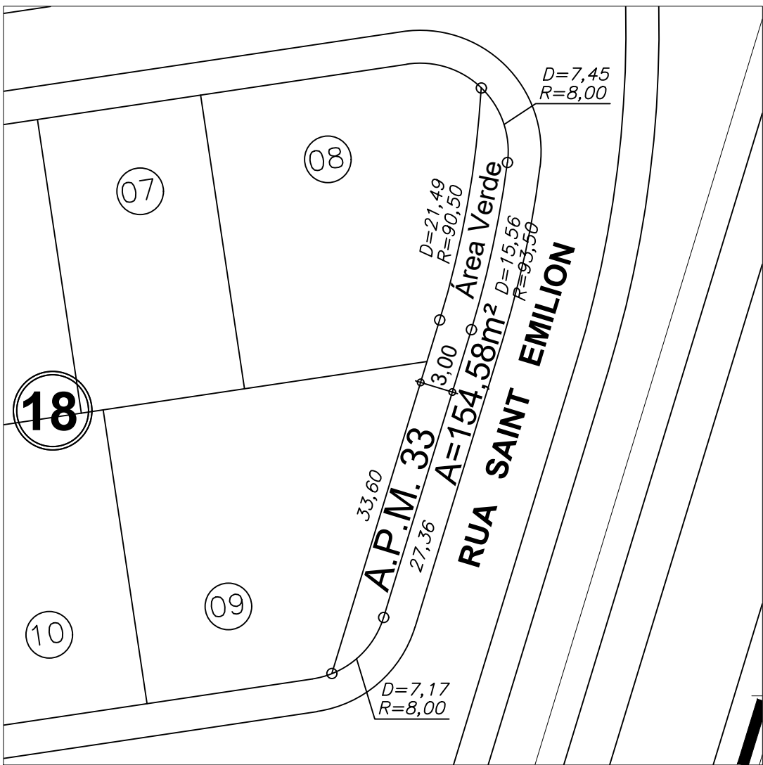
DETALHE DA A.P.M.V. 33 Esc: 1:500
