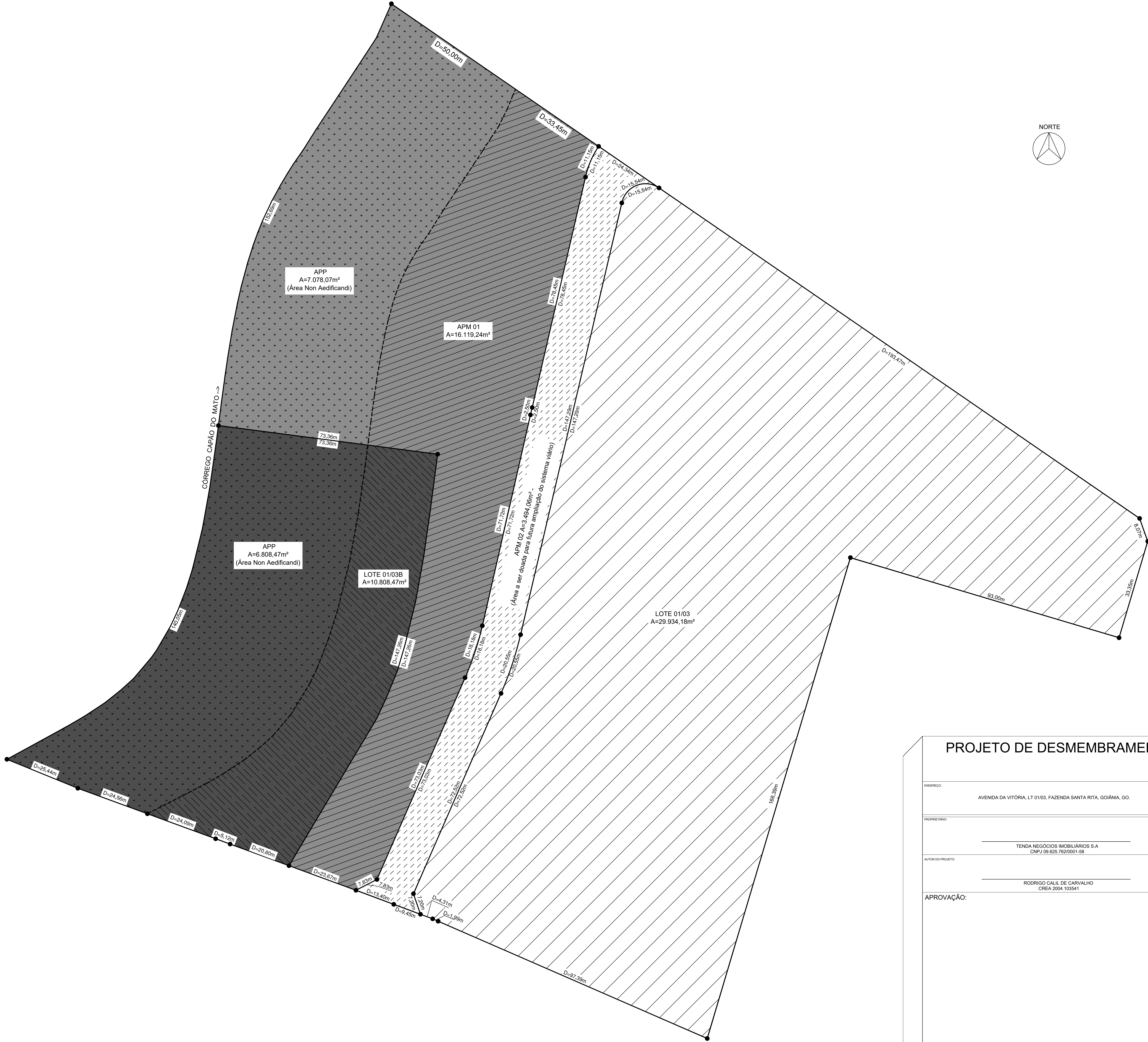
DESMEMBRAMENTO PROPOSTO ESC. 1:500
