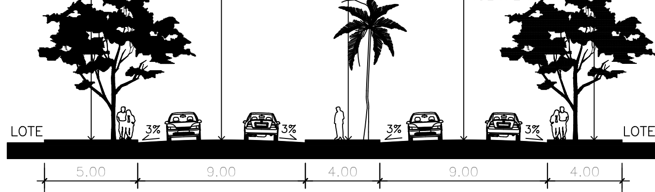
SEÇÃO TRANSVERSAL DA AVENIDA MARGINAL LESTE esc.: 1:200
