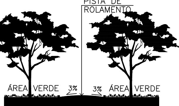
SEÇÃO TRANSVERSAL DAS VIAS DE 4m esc.: 1:200
