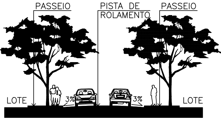
SEÇÃO TRANSVERSAL DAS VIAS DE 13m esc.: 1:200
