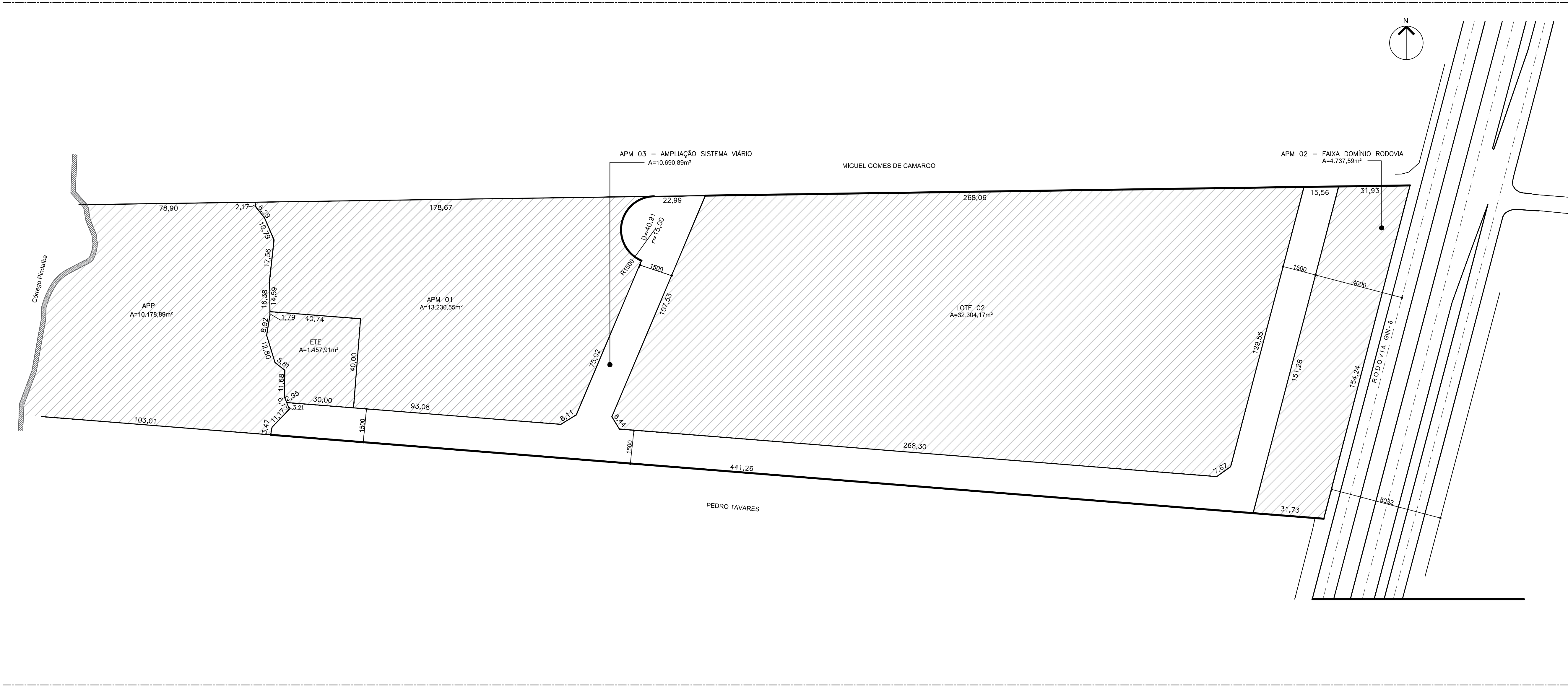
PLANTA DE SITUAÇÃO APÓS DESMEMBRAMENTO ESCALA 1:1000
