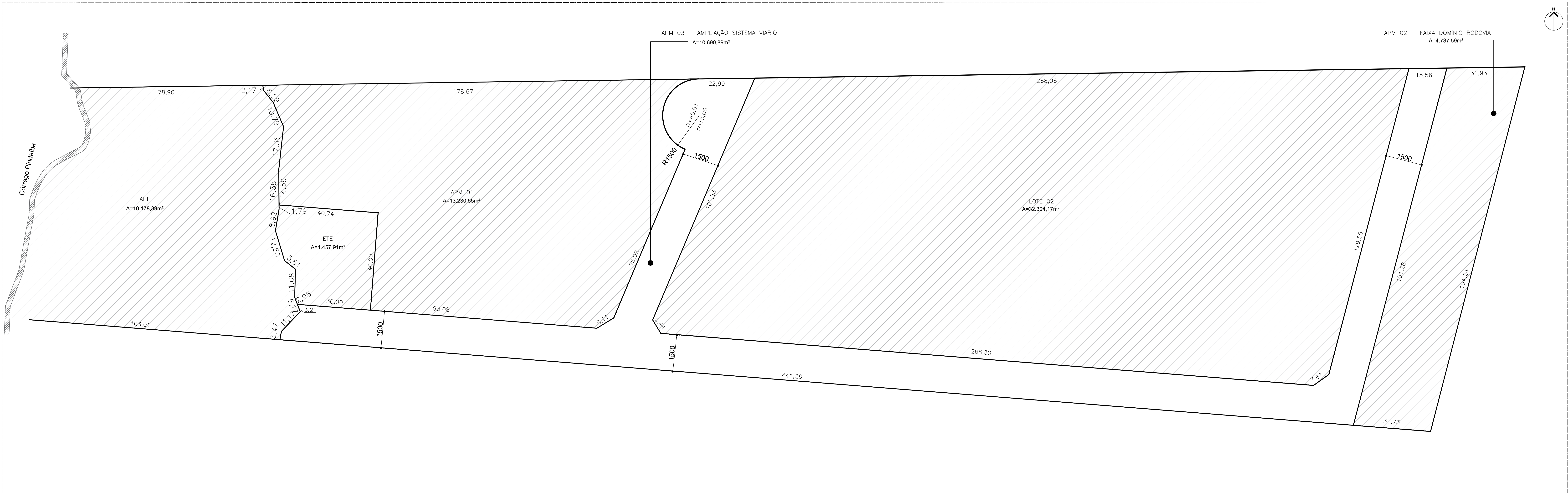
PLANTA DE DESMEMBRAMENTO PROPOSTO ESCALA 1:500
