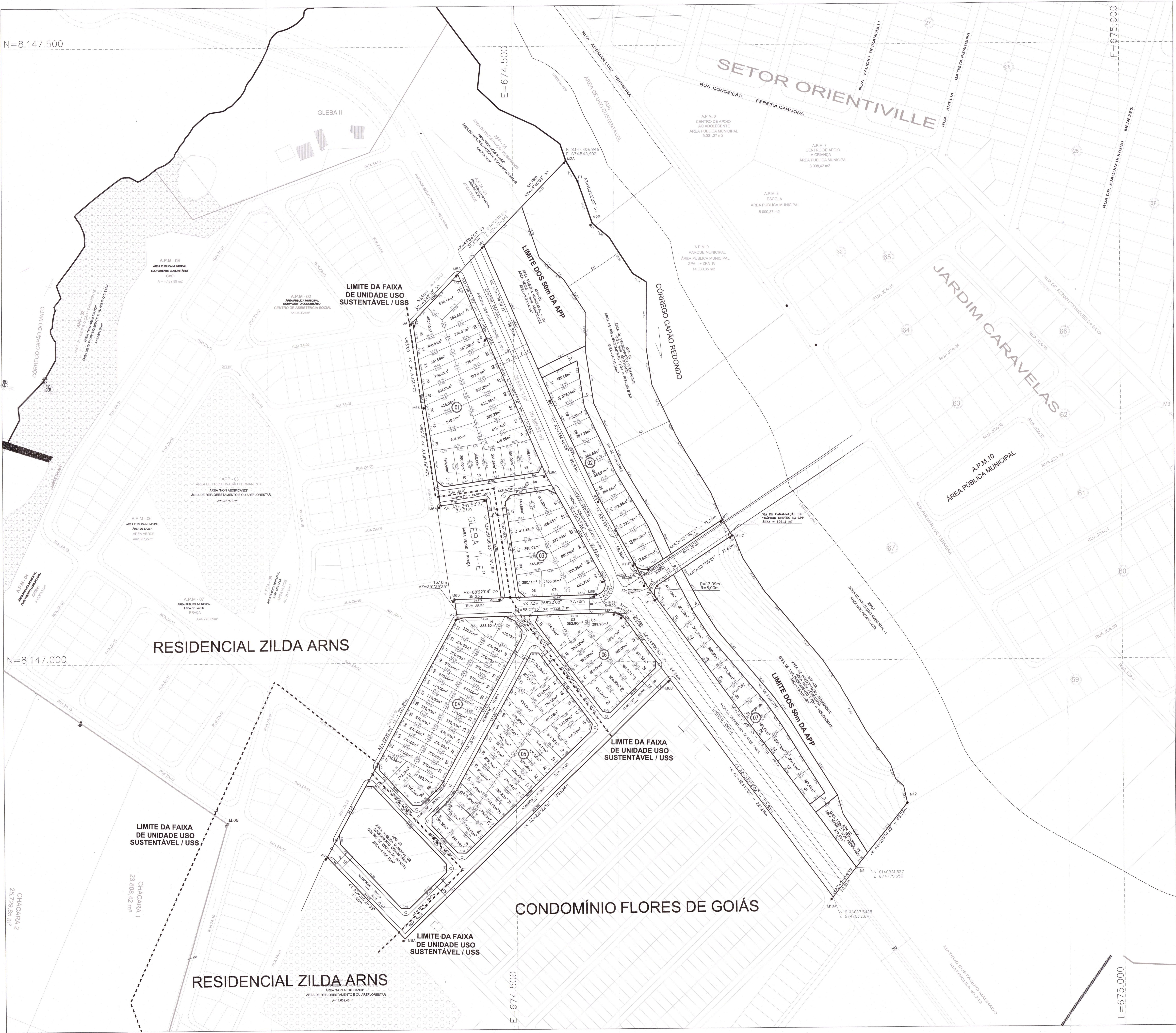
PLANTA CADASTRAL Escala 1:5000
