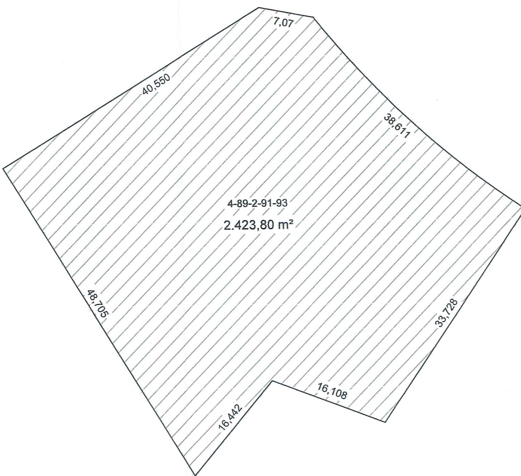
02 REMEMBRAMENTO PROPOSTO ESCALA 1:500
