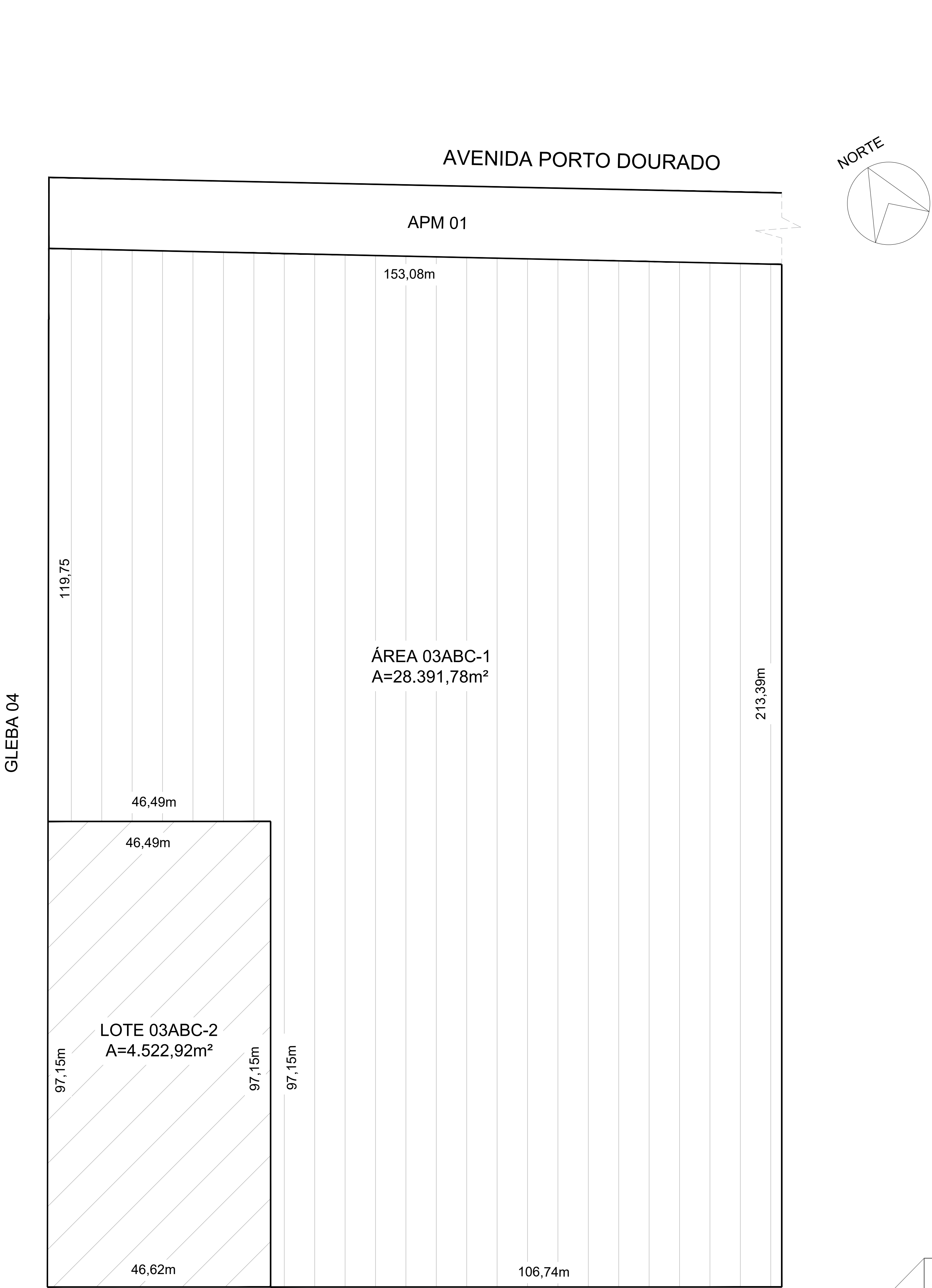
DESDOBRO PROPOSTO ESC. 1/1000
